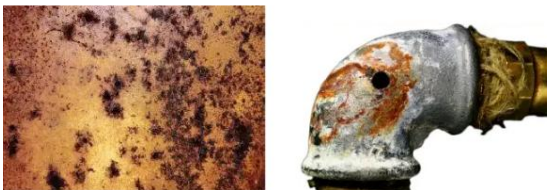
Figura 2: Corrosión localizada -Pitting (Zavaleta, 2019)
