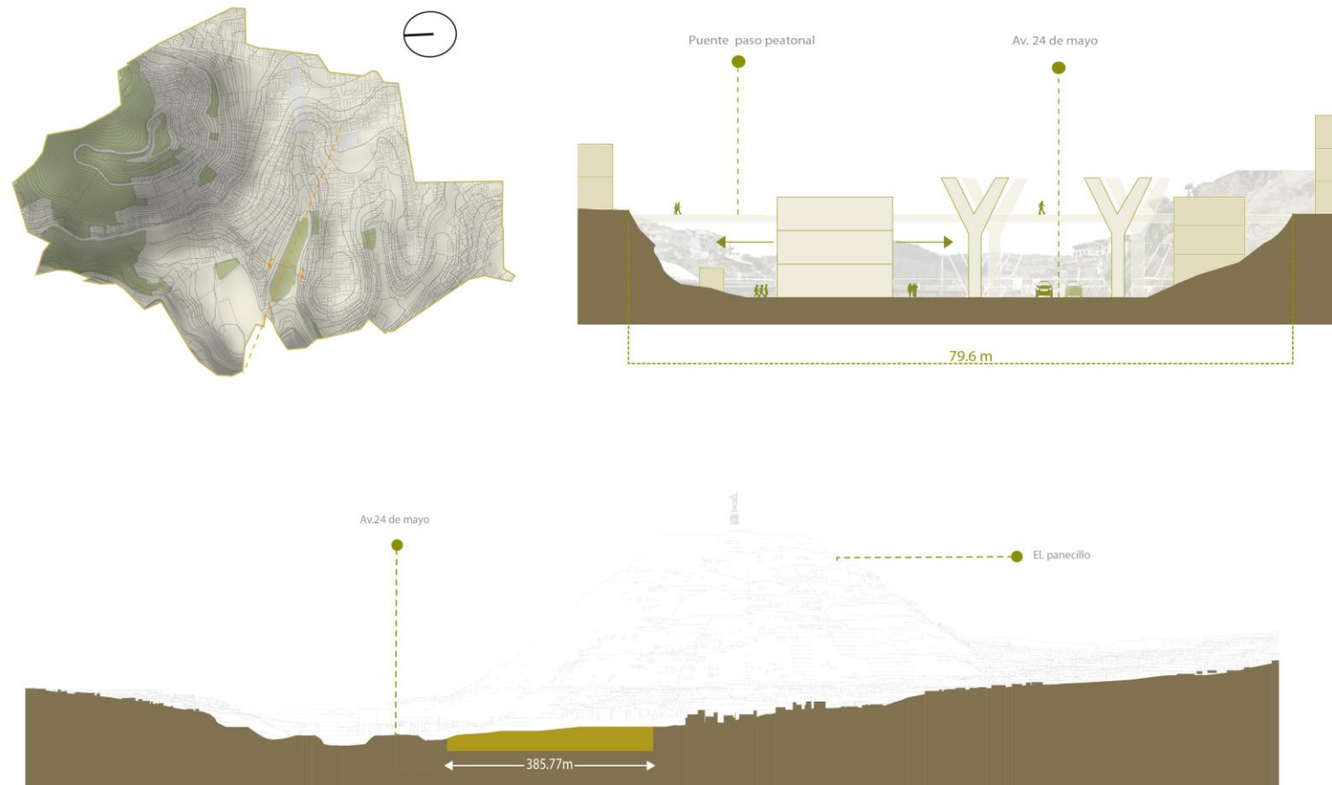
Figura 46 Topografía y corte contexto urbano del PUC
